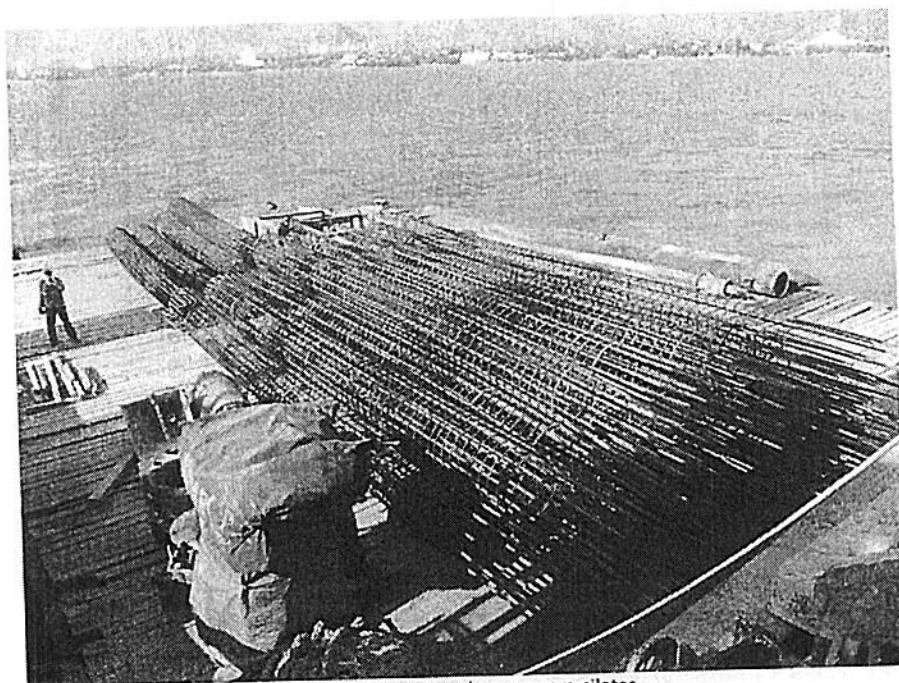
Foto 12. Estructura de acero para pilotes.
