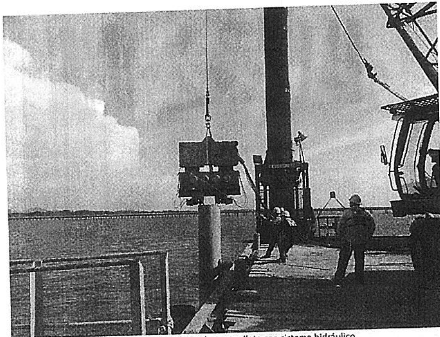
Foto 11. Instalación de tubo para pilote con sistema hidráulico.
