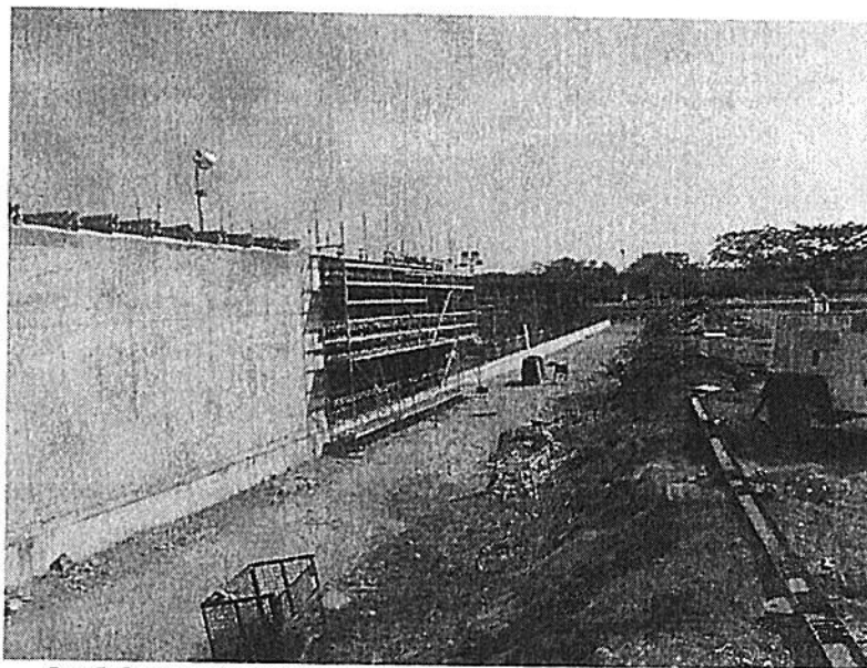
Foto 5. Construcción de túnel en concreto en área para almacenamiento de carbón.
