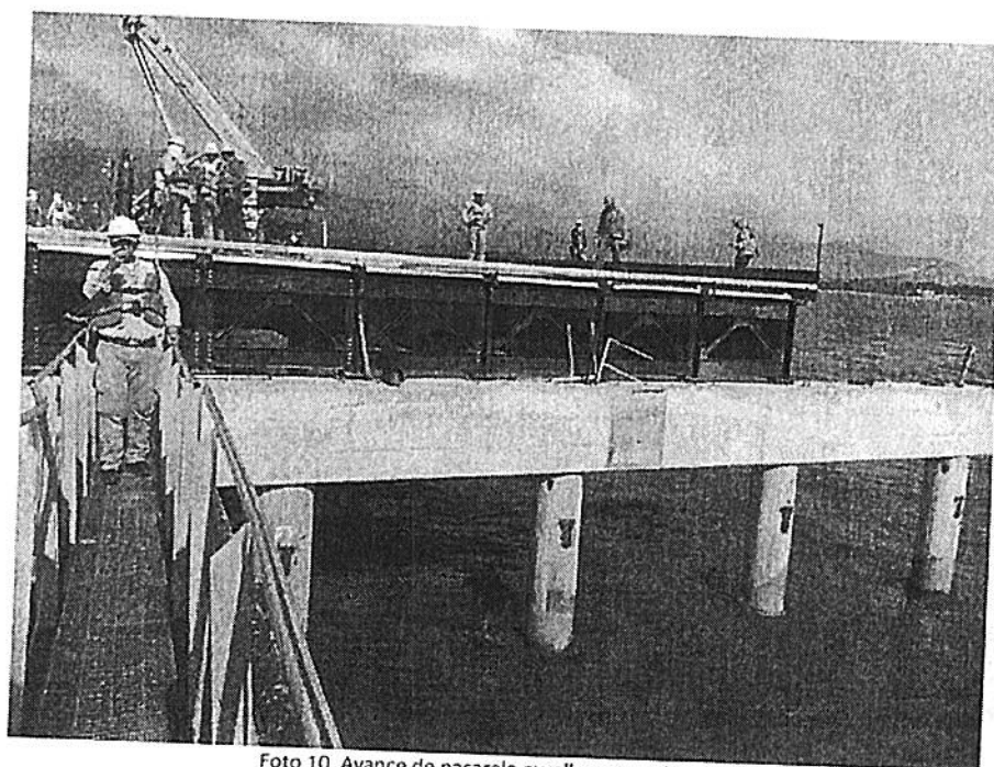
Foto 10. Avance de pasarela muelle cargue directo.
