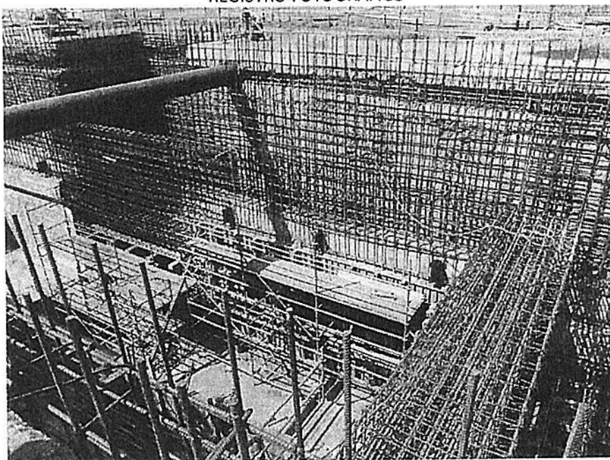
Foto 1. Construcción de volteador (car dumper cuádruple) para descargue de trenes.
