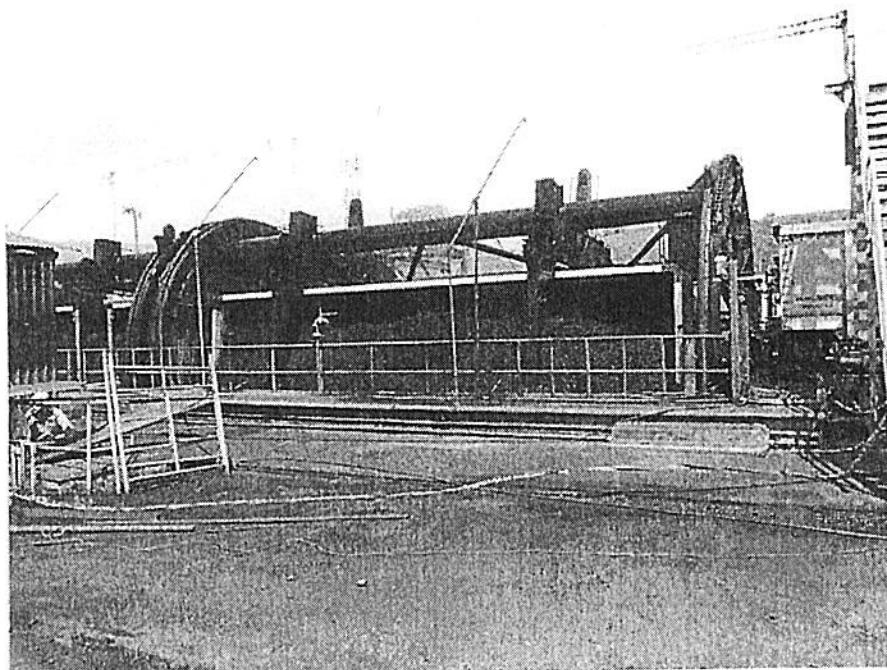
Foto 2. Sistema de descargue de trenes actual (Car dumper doble).
