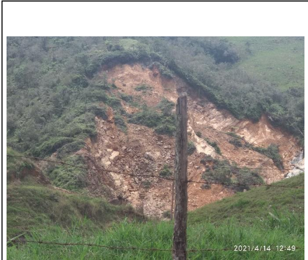
Foto 1: Corona de deslizamiento
